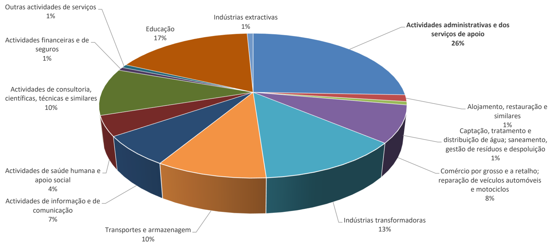
Gráfico 3 - Avisos prévios de greve por CAE (março 2024)
